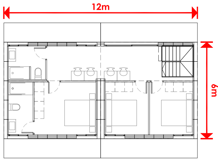
PLANTA PRIMERA
