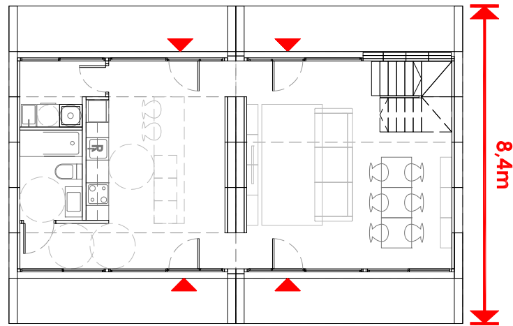
PLANTA BAJA
